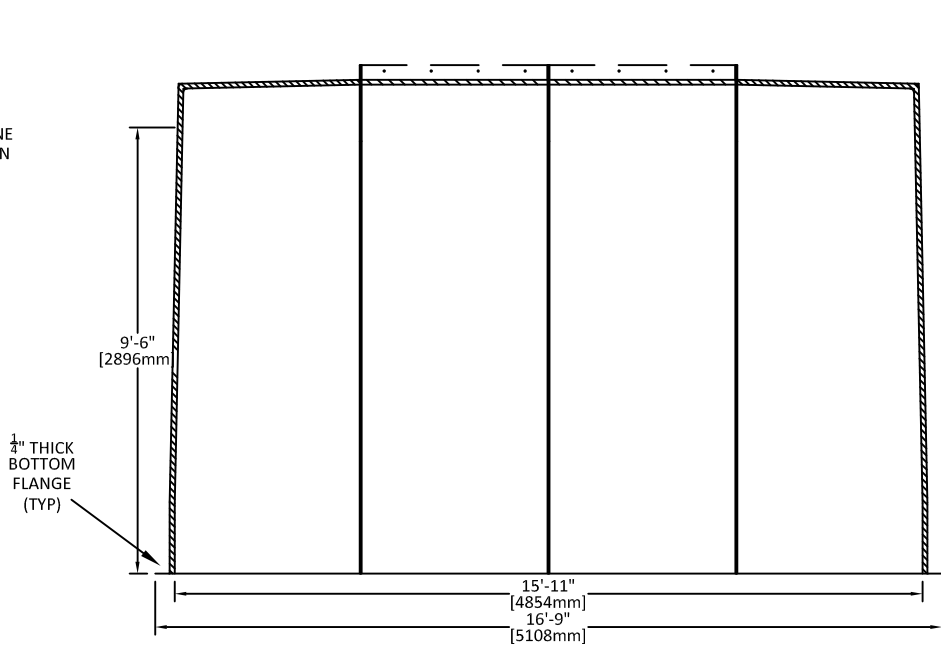
RIGHT ELEV.
