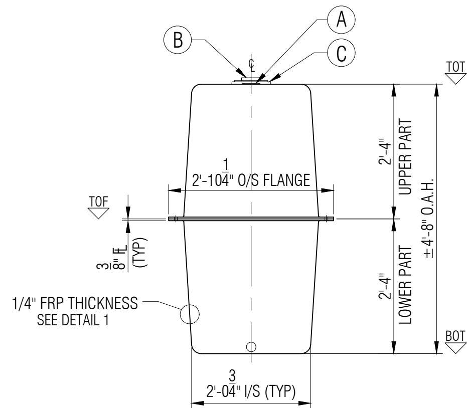
ELEVATION A
