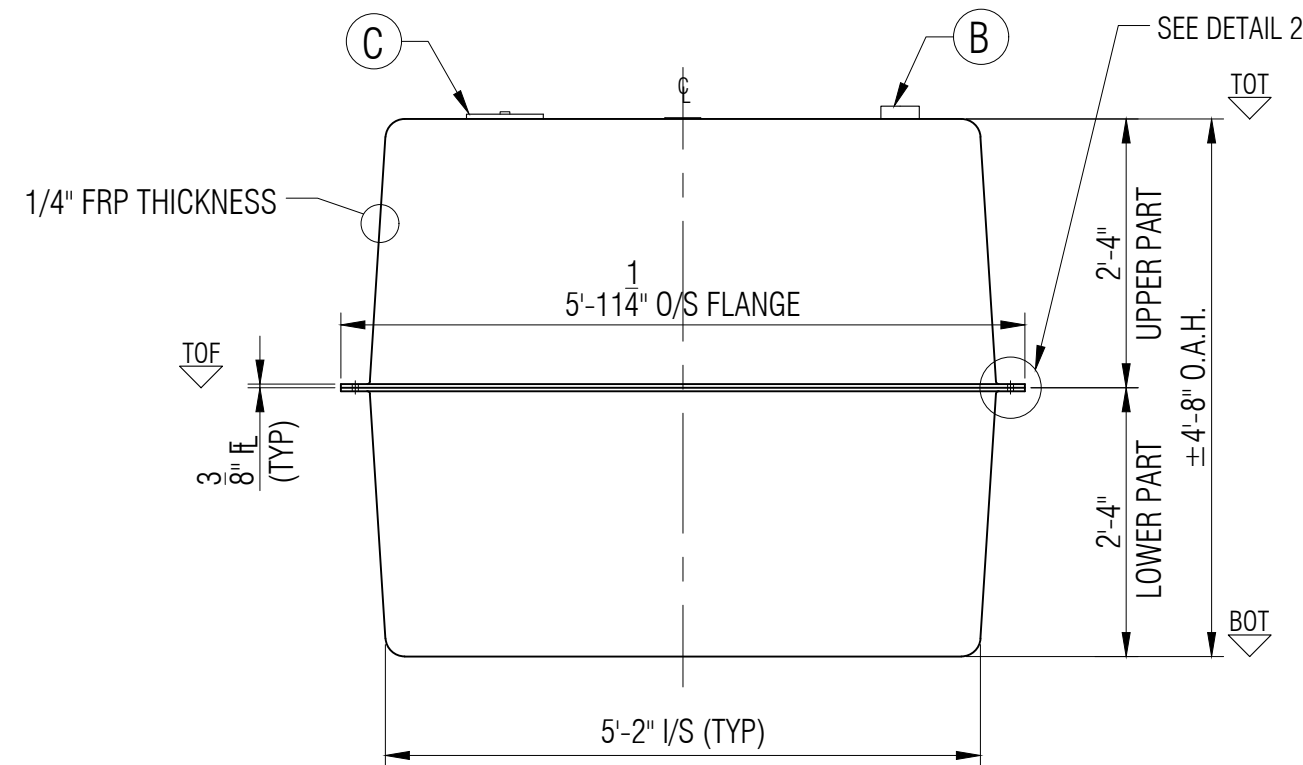
ELEVATION B
