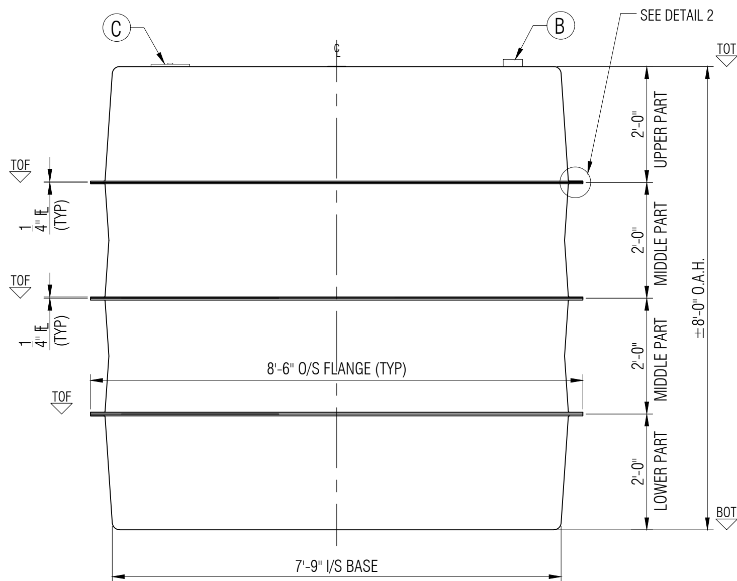
ELEVATION A
