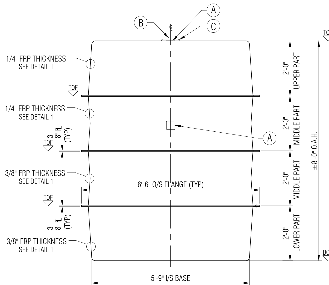
ELEVATION B
