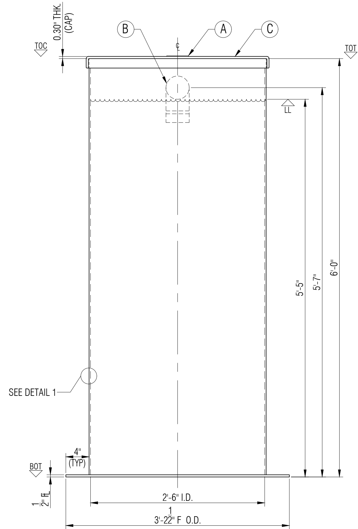
ELEVATION B
