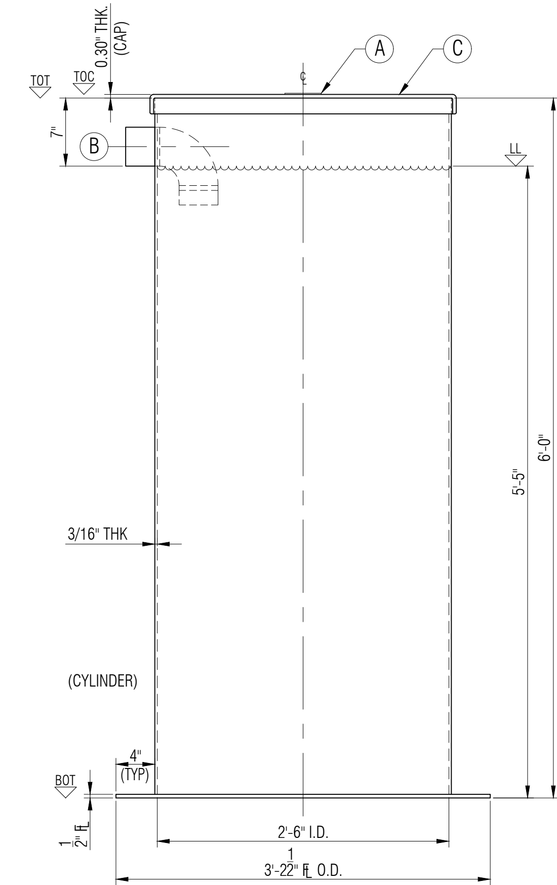
ELEVATION A
