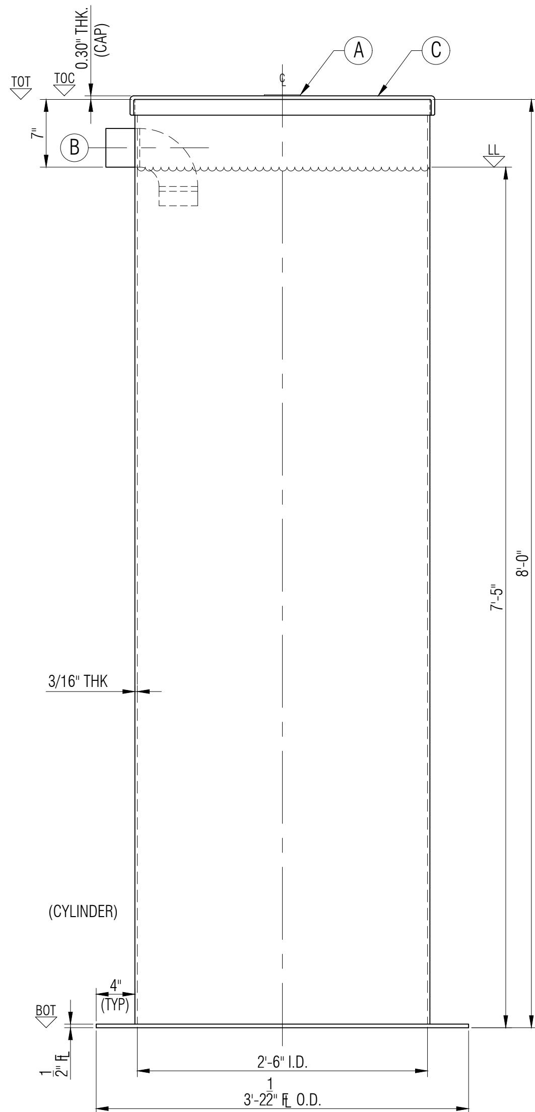
ELEVATION A
