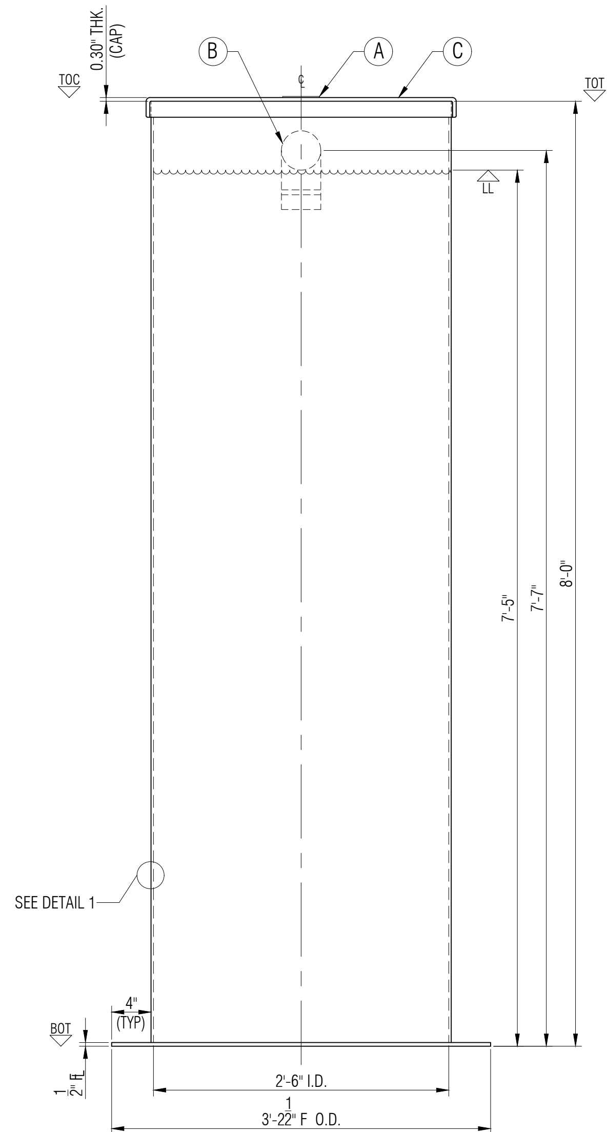
ELEVATION B
